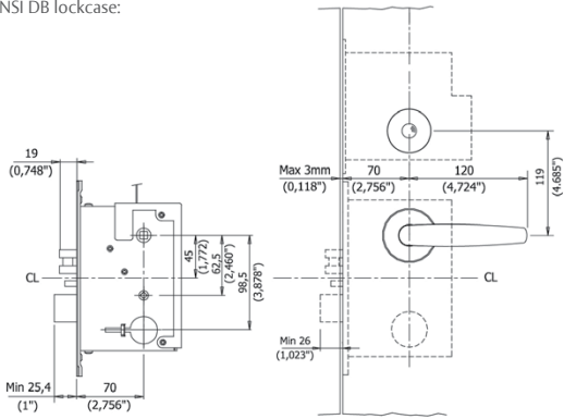
ANSI DB lockcase:
