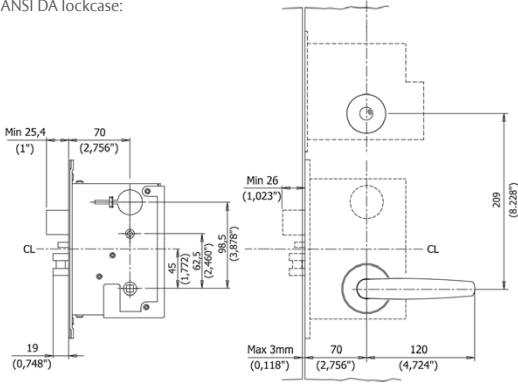
ANSI DA lockcase:
